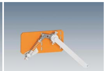
Lage des Spannschlüssels in Reinigungsposition
